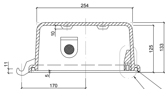
SECCIÓN B-B
