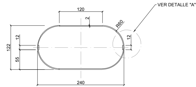
DETALLE TUBO PEANA
