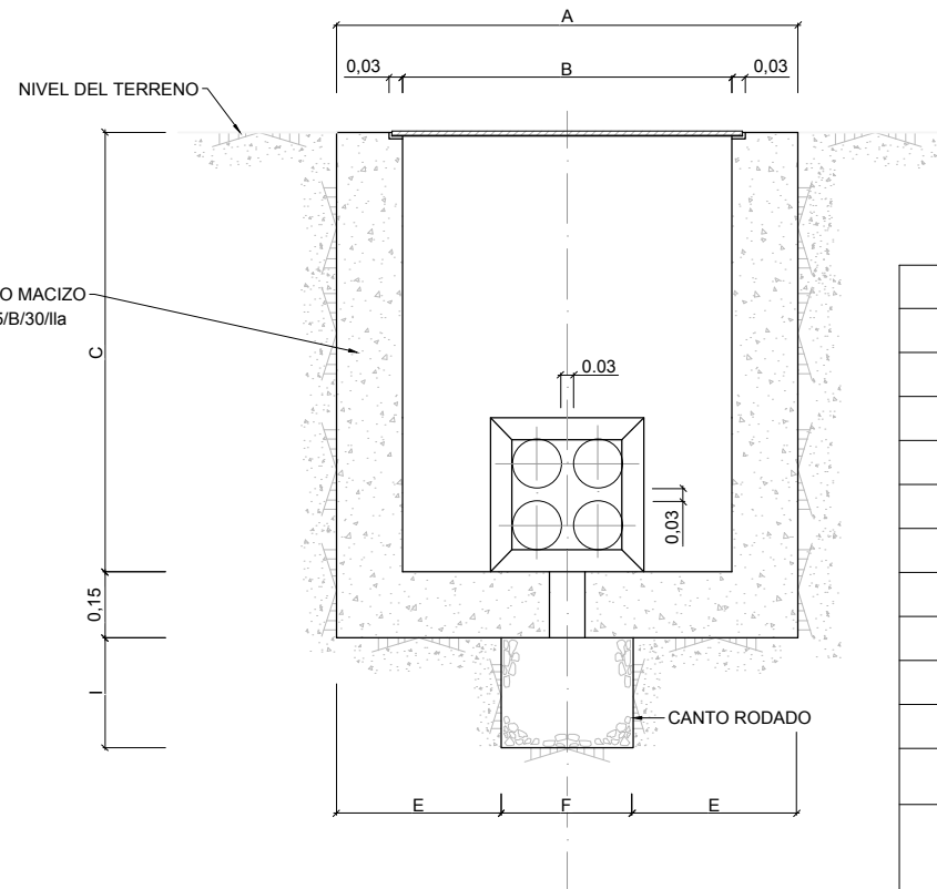
SECCIÓN TRANSVERSAL
