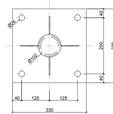
DETALLE COLUMNA
