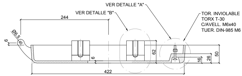
SECCIÓN A-A
