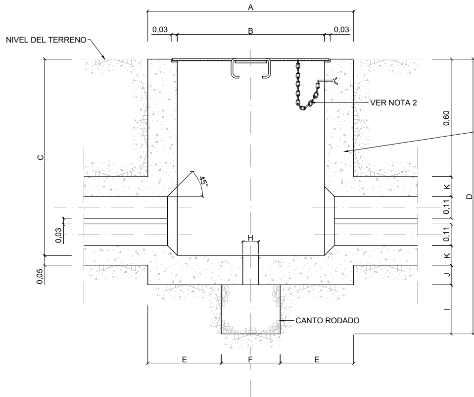
SECCIÓN LONGITUDINAL
