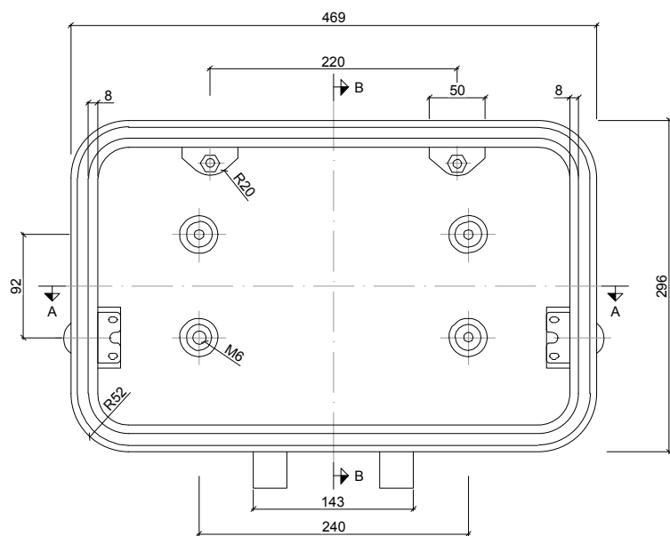
VISTA INFERIOR
