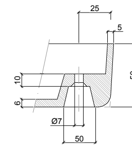
DETALLE "A"
