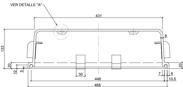
SECCIÓN A-A
