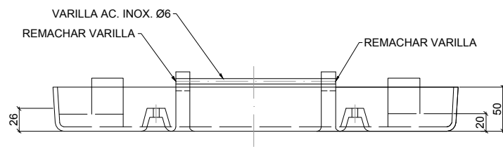
VISTA POSTERIOR
