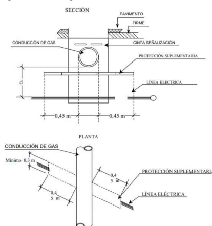
Figura 3. Cruzamiento con canalizaciones de gas
