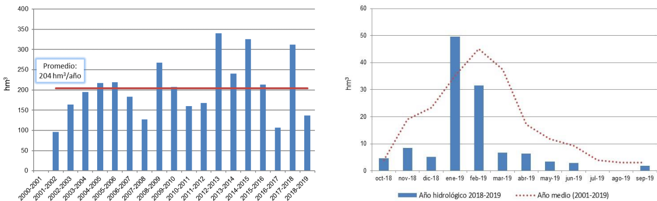
Figura 14 Evolución de la aportación en la estación Sodaupé (Fuente: Diputación Foral de Bizkaia) 1
