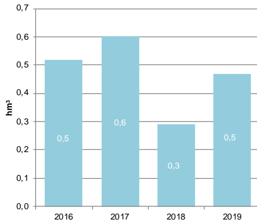
Figura 46 Evolución de la reutilización de agua en la EDAR de Zuringoain (Fuente: Consorcio de Aguas de Gipuzkoa)
