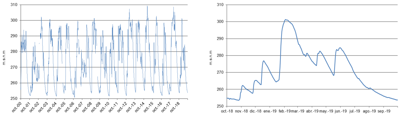
Figura 31 Evolución de niveles en la estación DTH-1 (Fuente: Agencia Vasca del Agua-Diputación Foral de Gipuzkoa)
