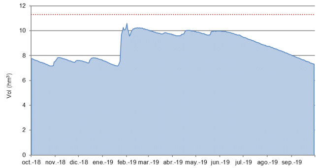
Figura 39 Evolución de volúmenes en el embalse de Ibaieder (Fuente: Consorcio de Aguas de Gipuzkoa)
