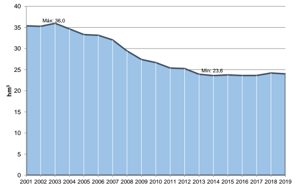
Figura 53 Volumen suministrado por Aguas del Añarbe (Fuente: Aguas del Añarbe)
