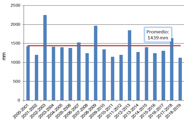
Figura 6 Evolución de la precipitación de la estación de Berriatua (Fuente: Euskalmet)
