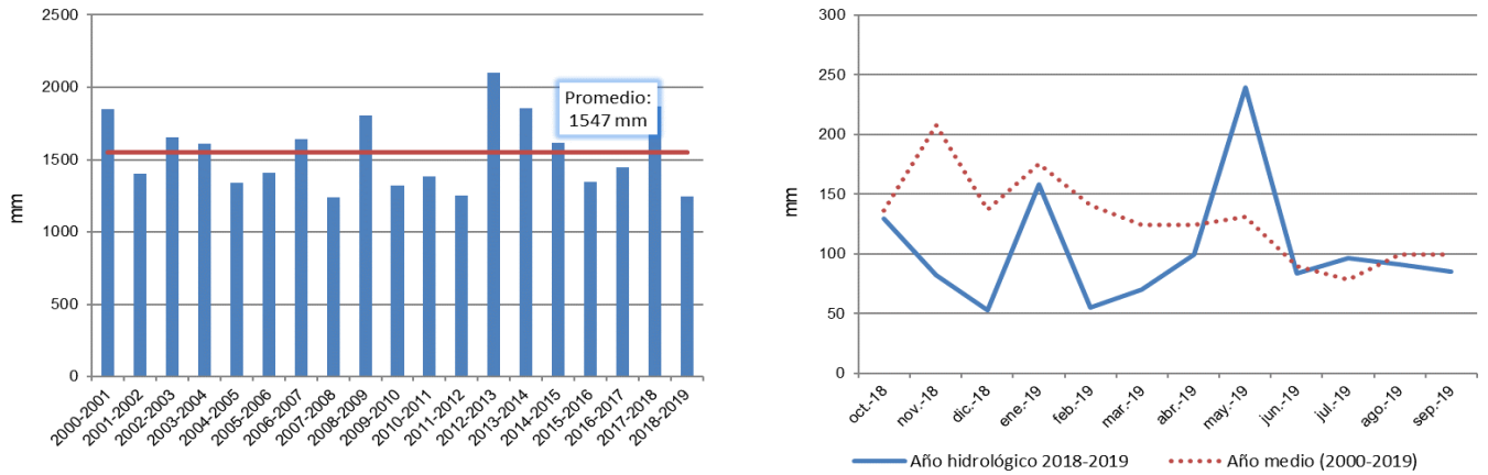
Figura 8 Evolución de la precipitación de la estación de Oiartzun (Fuente: Euskalmet)
