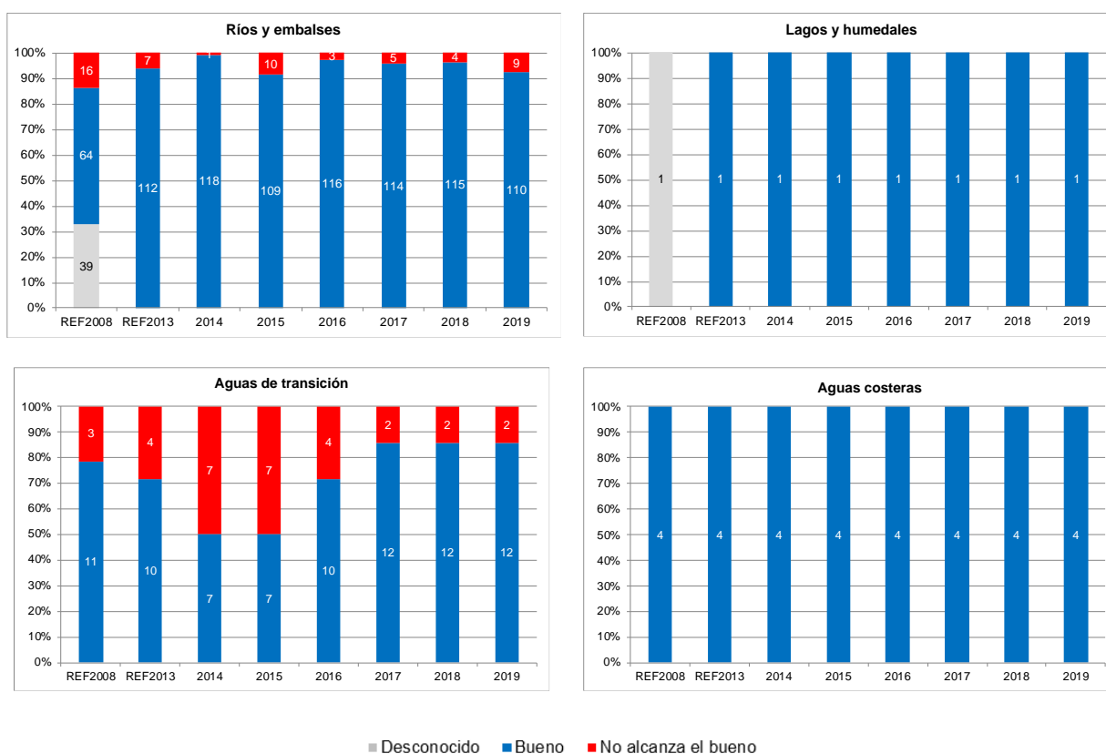
Figura 72 Evolución del estado químico de las masas de agua superficial
