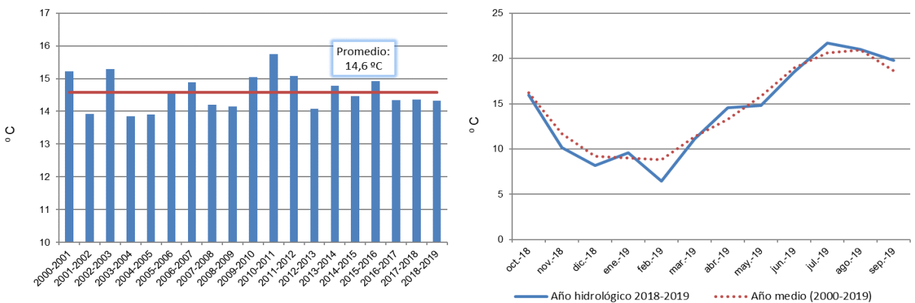
Figura 11 Evolución de la temperatura de la estación de Altzola (Fuente: Euskalmet)
