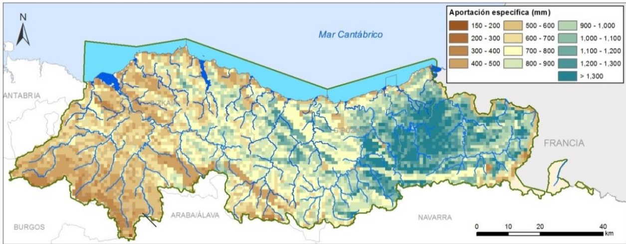
Figura 13 Aportación media en la demarcación
