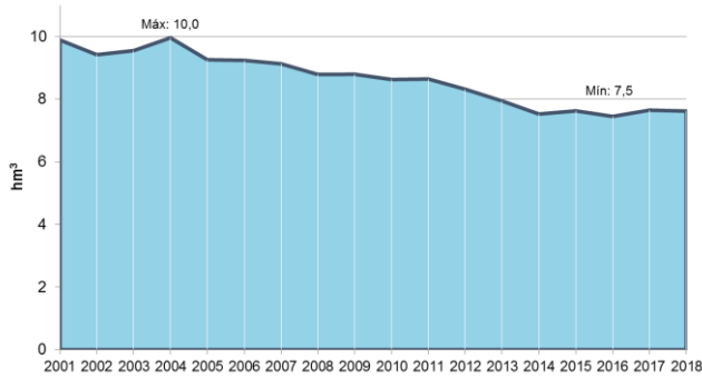
Figura 54 Volumen de entrada a la ETAP de Elordi (Fuente: Servicios de Txingudi)
