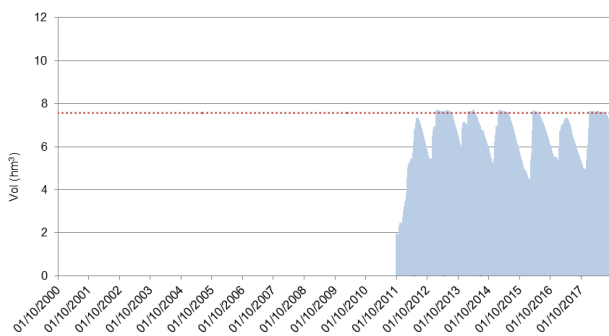
Figura 43 Evolución de volúmenes en el embalse de Ibiur (Fuente: Consorcio de Aguas de Gipuzkoa)
