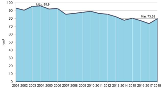
Figura 52 Volumen suministrado desde la ETAP de Venta Alta (Fuente: Consorcio de Aguas Bilbao Bizkaia)
