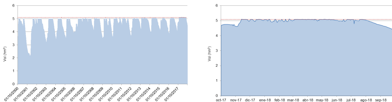
Figura 45 Evolución de volúmenes en el embalse de San Antón (Fuente: Servicios de Txingudi, S.A.)
