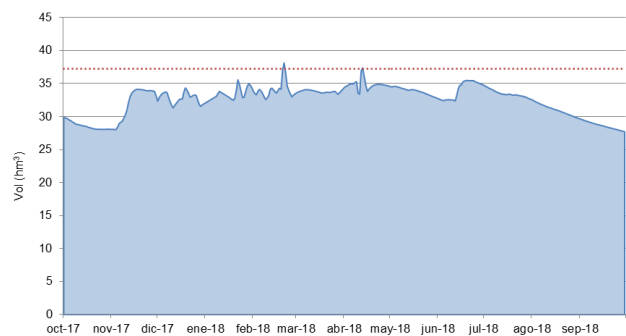
Figura 44 Evolución de volúmenes en el embalse de Añarbe (Fuente: Confederación Hidrográfica del Cantábrico – Agencia Vasca del Agua)
