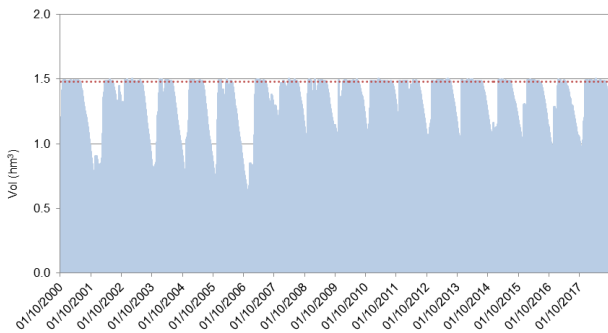
Figura 39 Evolución de volúmenes en el embalse de Urkulu (Fuente: Consorcio de Aguas de Gipuzkoa)
