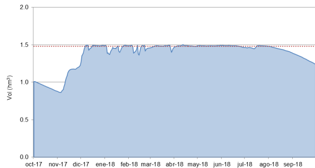
Figura 39 Evolución de volúmenes en el embalse de Urkulu (Fuente: Consorcio de Aguas de Gipuzkoa)
