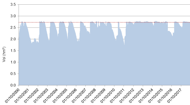
Figura 37 Evolución de volúmenes en el embalse de Ordunte (Fuente: Confederación Hidrográfica del Cantábrico-Agencia Vasca del Agua)
