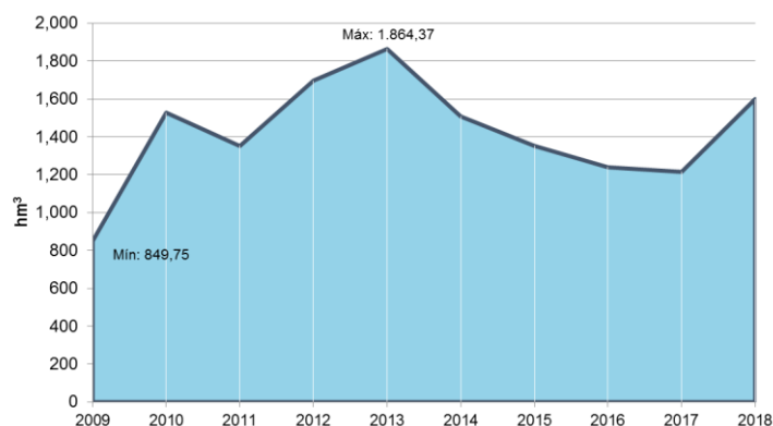
Figura 61 Volumen turbinado (Fuente: Canon del agua de la CAPV)
