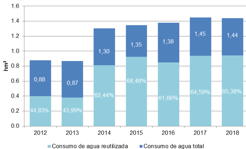
Figura 47 Evolución de la reutilización de agua en la EDAR de Galindo (Fuente: Consorcio de Aguas Bilbao Bizkaia)
