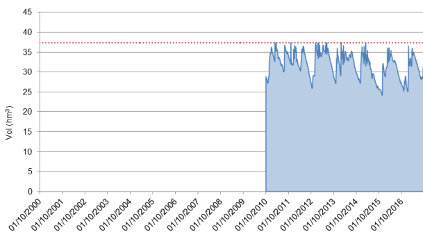
Figura 44 Evolución de volúmenes en el embalse de Añarbe (Fuente: Confederación Hidrográfica del Cantábrico)
