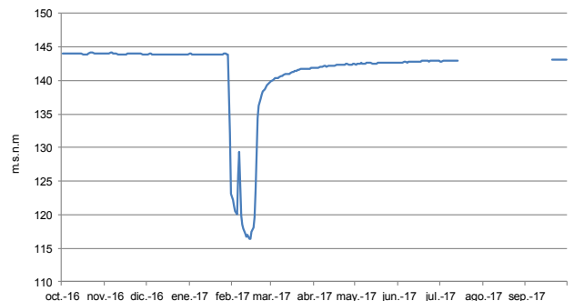
Figura 35 Evolución de niveles en la estación Elduaien-3 (Fuente: Agencia Vasca del Agua-Diputación Foral de Gipuzkoa)
