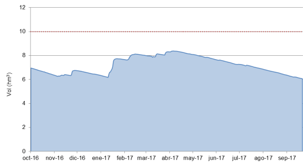
Figura 43 Evolución de volúmenes en el embalse de Ibiur (Fuente: Consorcio de Aguas de Gipuzkoa)
