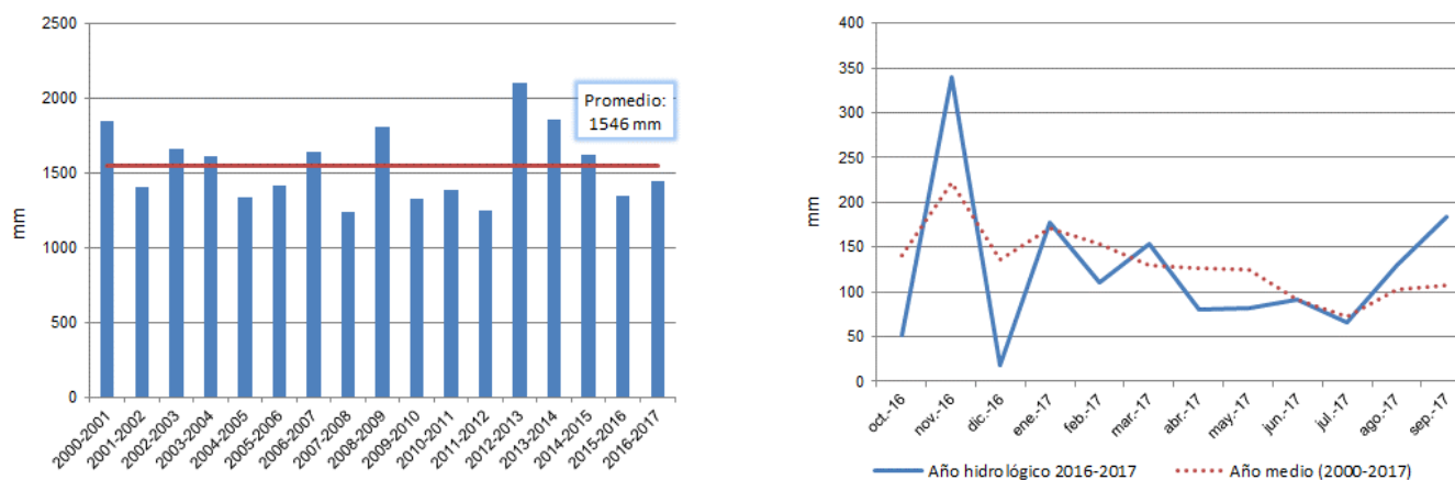
Figura 8 Evolución de la precipitación de la estación de Alzola (Fuente: Euskalmet)
