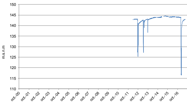
Figura 35 Evolución de niveles en la estación Elduaien-3 (Fuente: Agencia Vasca del Agua-Diputación Foral de Gipuzkoa)
