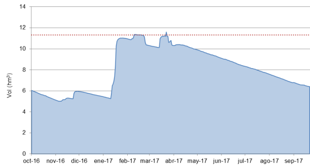
Figura 41 Evolución de volúmenes en el embalse de Arriaran (Fuente: Consorcio de Aguas de Gipuzkoa)
