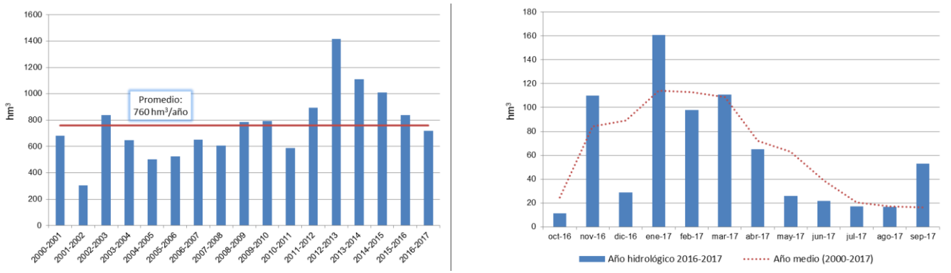
Figura 28 Evolución de la aportación en la estación Enderlatza (Fuente: Confederación Hidrográfica del Cantábrico)
