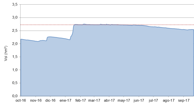
Figura 37 Evolución de volúmenes en el embalse de Ordunte (Fuente: Confederación Hidrográfica del Cantábrico-Agencia Vasca del Agua)
