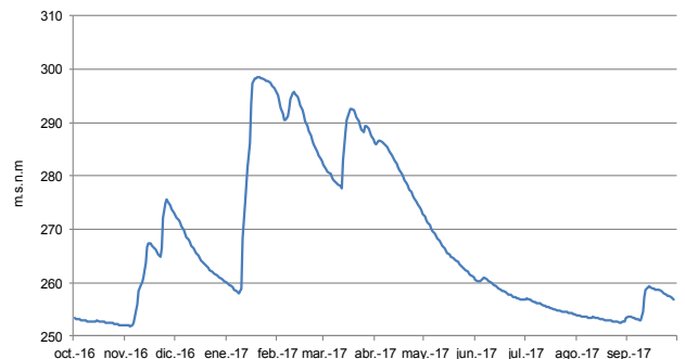
Figura 34 Evolución de niveles en la estación DTH-1 (Fuente: Agencia Vasca del Agua-Diputación Foral de Gipuzkoa)
