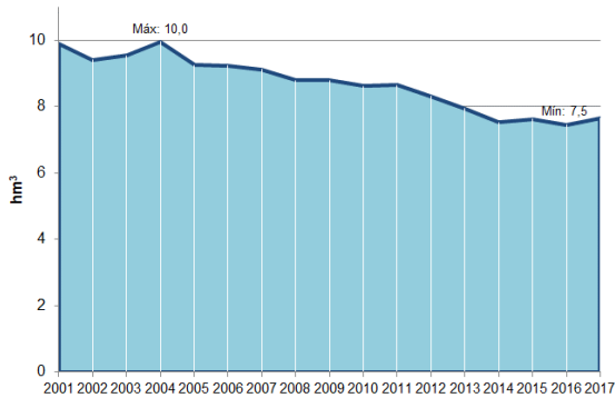
Figura 54 Volumen de entrada a la ETAP de Elordi (Fuente: Servicios de Txingudi)
