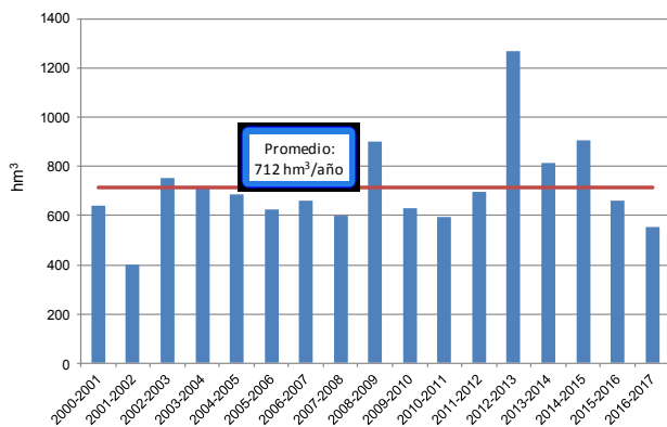
Figura 25 Evolución de la aportación en la estación Lasarte (Fuente: Diputación Foral de Gipuzkoa)
