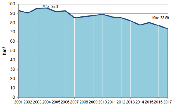
Figura 52 Volumen suministrado desde la ETAP de Venta Alta (Fuente: Consorcio de Aguas Bilbao Bizkaia)
