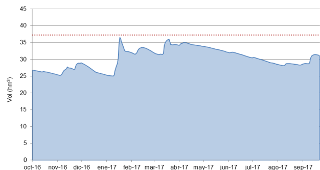
Figura 44 Evolución de volúmenes en el embalse de Añarbe (Fuente: Confederación Hidrográfica del Cantábrico)
