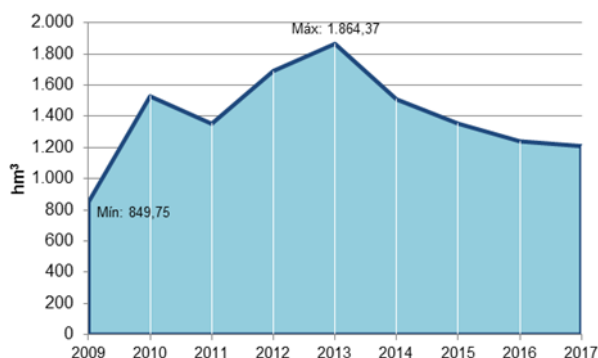
Figura 61 Volumen turbinado (Fuente: Canon del agua de la CAPV)
