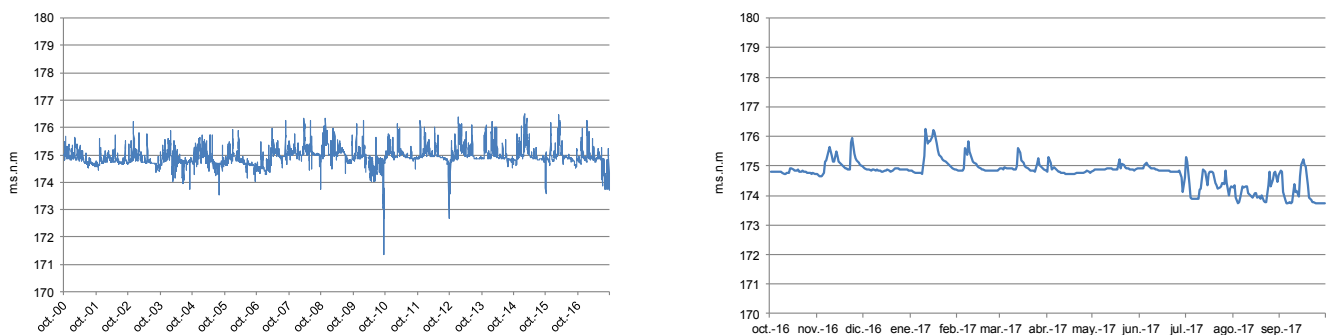
Figura 29 Evolución de niveles en la estación Mañaria-2 (Fuente: Agencia Vasca del Agua)
