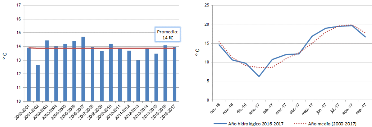
Figura 12 Evolución de la temperatura de la estación de Abusu (Fuente: Euskalmet)
