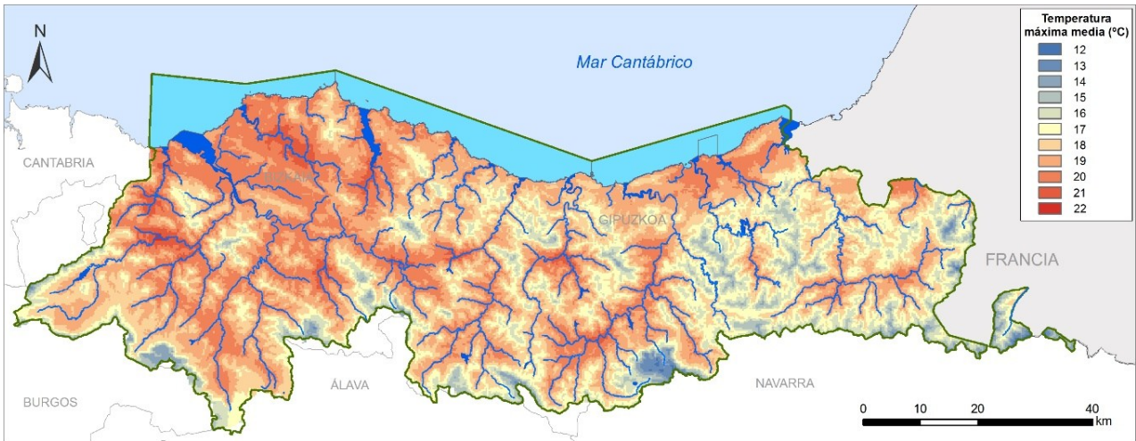
Figura 10 Temperatura máxima media en la demarcación
