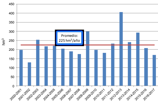
Figura 23 Evolución de la aportación en la estación Altzola (Fuente: Diputación Foral de Gipuzkoa)
