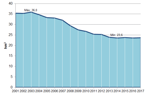
Figura 55 Volumen suministrado por Aguas del Añarbe (Fuente: Aguas del Añarbe)
